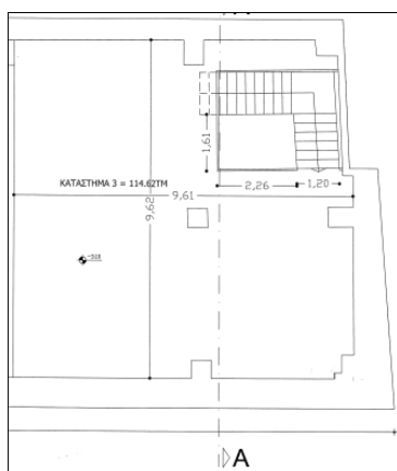
Κατόψη Υπογείου
