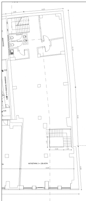
Κατόψη Παταριού
